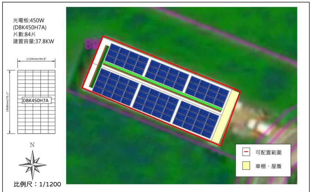
圖五、太陽光電設備規劃圖
